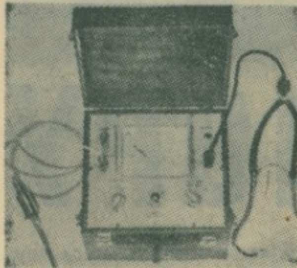
ОВАЈ ОДИМЕТАР ОМОГУЋАВА ДА СЕ УХВАТИ ШУМ ИЛИ ВИБРАЦИЈА КОЈУ СТВАРА НЕКИ ЕЛЕКТРИЧНИ АПАРАТ НАЗВАН ЕЛЕКТРИЧНО ЊУШКАЛО
