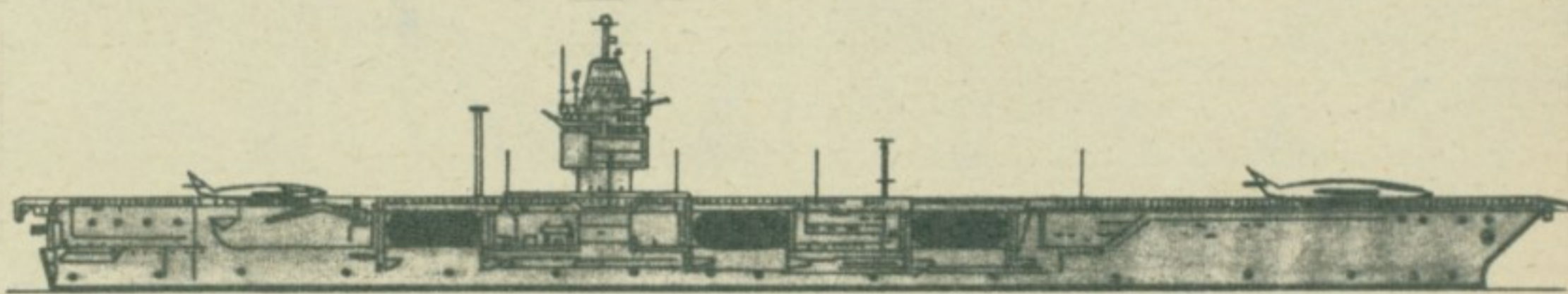
АМЕРИЧКИ ТЕШКИ НОСАЧ АВИОНА „ЕНТЕРПРАЈЗ“ поринут 1960, завршен 1961, депласман 83.500 т, дужина 317 м, ширина 76 м, газ 7,6 м, површина узлетно-слетне палубе 317 x 70 м, носивост 100 авиона, брзина 35 чв (око 64 км/ч), посада 2870 морнара и око 2000 пилота и ваздухопловно-техничког особља.
