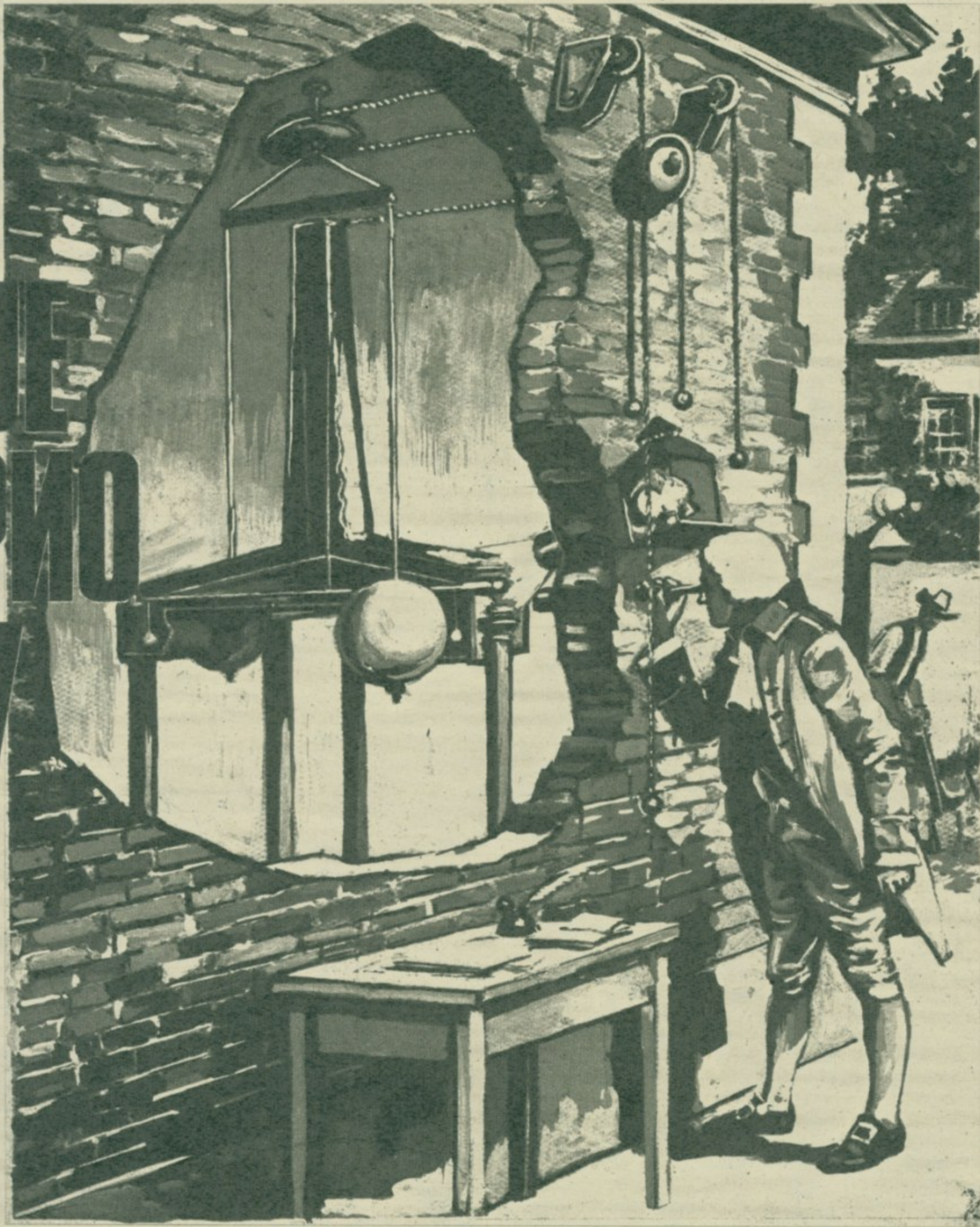
ДА БИ МЕРЕЊА БИЛА ШТО ТАЧНИЈА, КЕВЕНДИШ ЈЕ ЕКСПЕРИМЕНТ ПОСМАТРАО КРОЗ РУПУ У ЗИДУ ЛАБОРАТОРИЈЕ.
