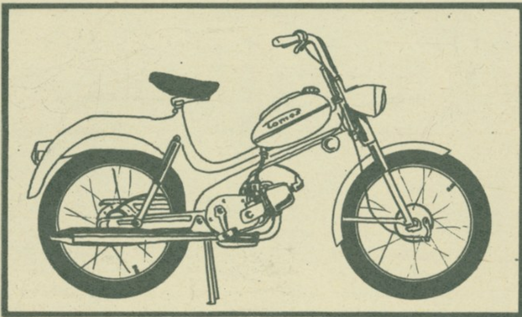
КОЛИБРИ АО-Н: 1,8 КС, највећа брзина 48 км на час, просечна потрошња горива 2,2 л на 100 км, резервоар 5,5 литара.
