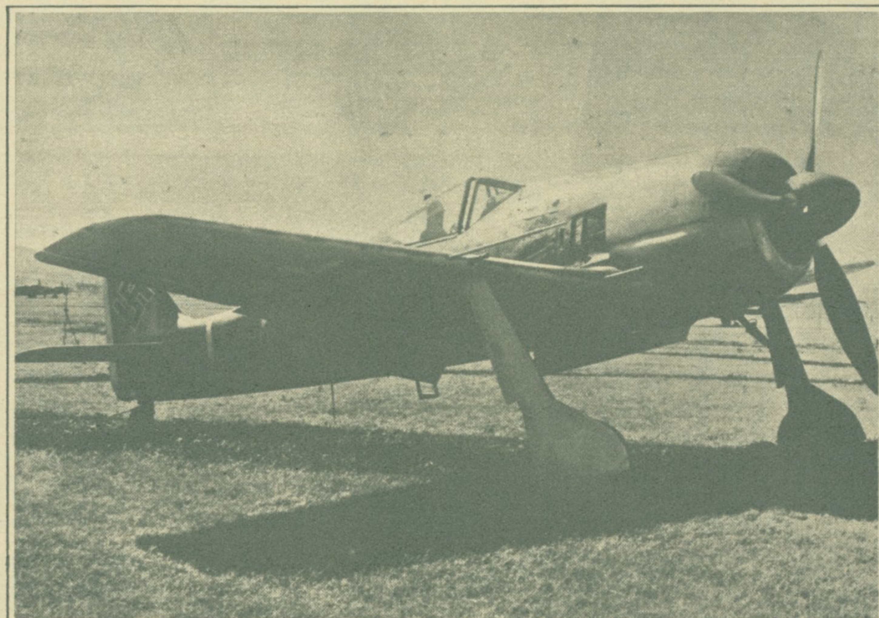
ФОКЕ-ВУЛФ 190 А: ловац једносед, металне конструкције, једнокрилац с мотором БМВ-801 од 1875 КС у звезди. Верзија Д има мотор Дајмлер Бенц од 2000 КС. Брзина 680 км/ч. Распон крила 10,50 м, дужина 8,84 м, тежина 4000 кг. Четири топа калибра 20 мм и два митраљеза калибра 13 мм.
