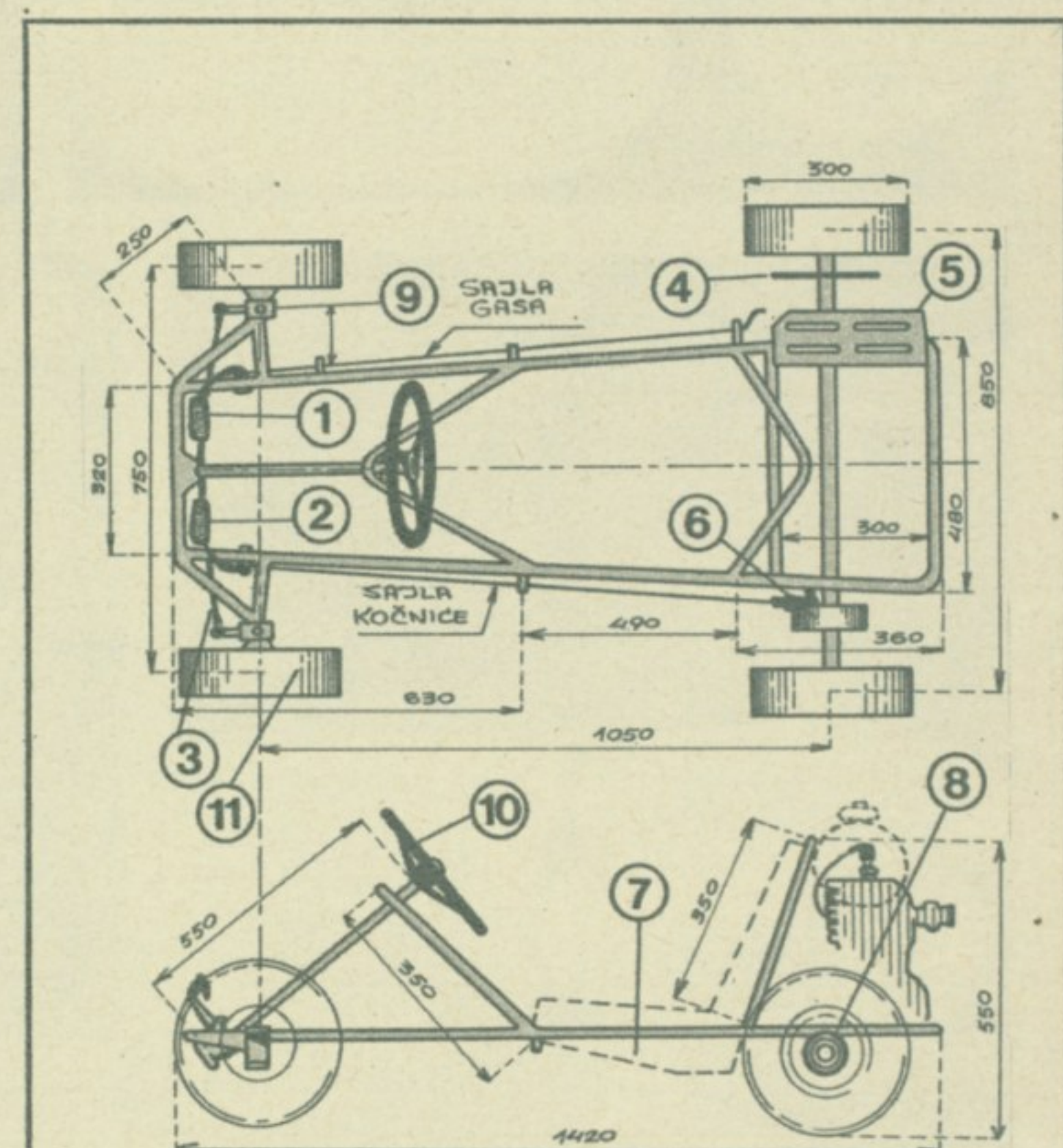
КАРТИНГ ЗА МОТОРЕ ОД 100 ССМ: 1. педала гаса, 2. педала кочнице, 3. систем за управљање, 4. ланчаник, 5. носач мотора, 6. добош кочница, 7. седиште, 8. погонска осовина, 9. зглоб управљача, 10. управљач, 11. точак.
