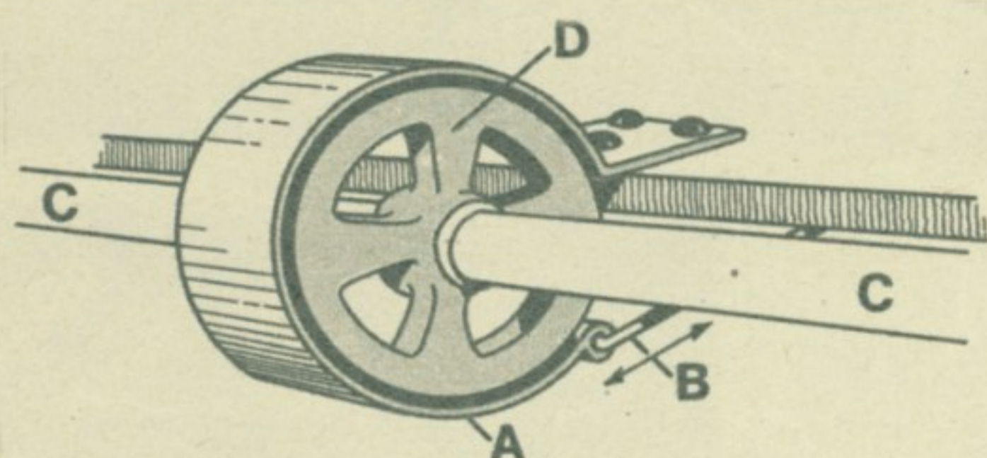
КОЧНИЦА: а) лим — облога, б) сајла — шипка, с) погонска осовина, д) добош кочнице.
