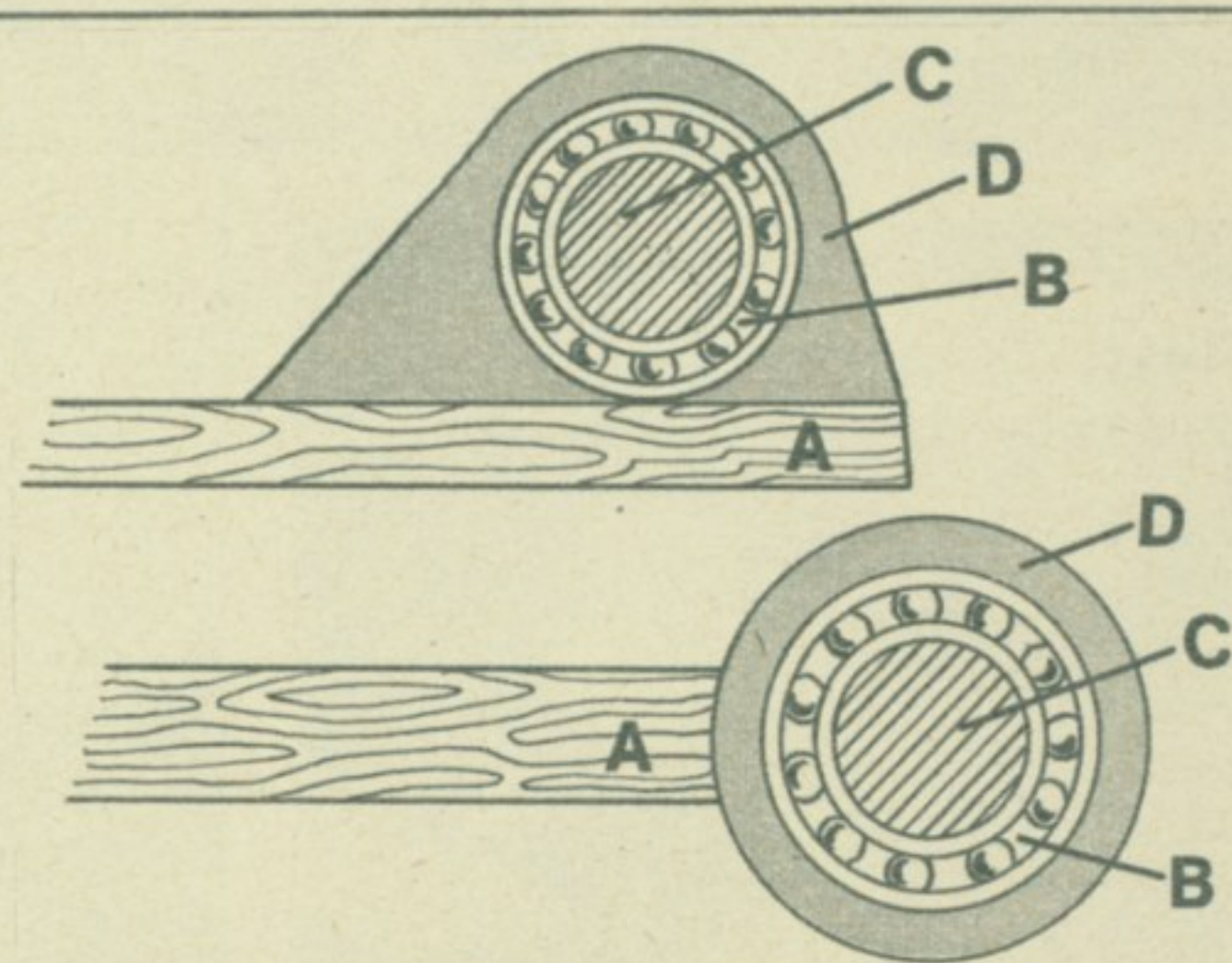
ЛЕЖАЈЕВИ ПОГОНСКЕ ОСОВИНЕ: а) шасија, б) лежај, с) погонска осовина, д) лим — држач лежачега (пример бр. 1); а) шасија, б) лежај, с) погонска осовина, д) носач лежачега (пример бр. 2).
