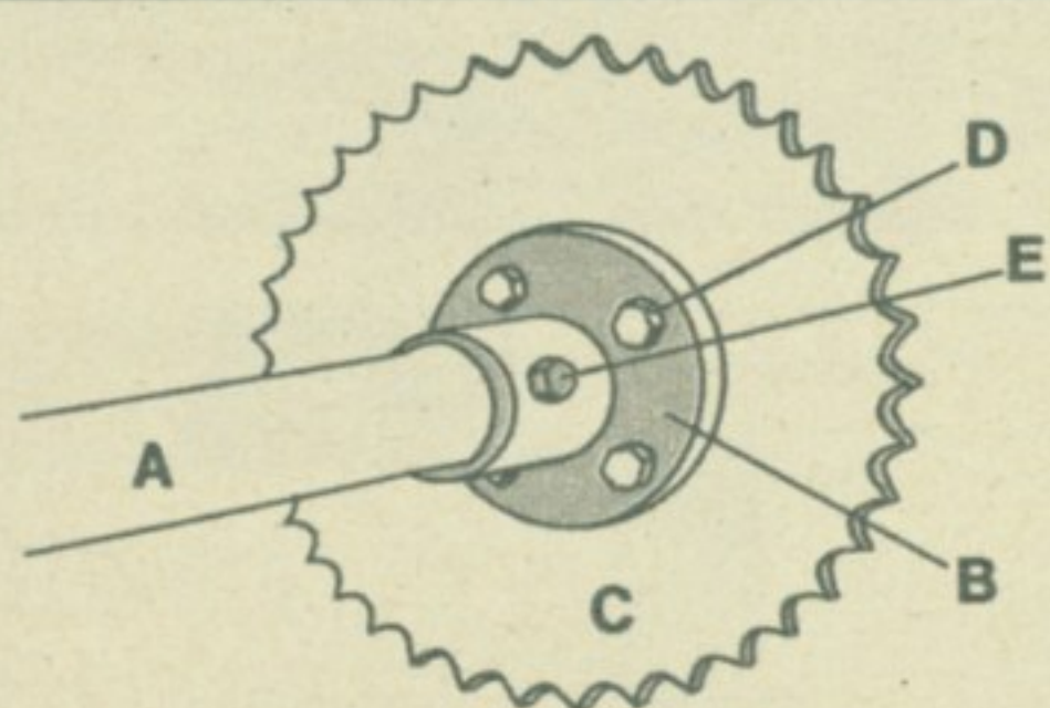
ЛАНЧАНИК (гледан из задњег левог угла): а) погонска осовина, б) причвршћивач ланчаника, с) ланчаник, д) шраф, е) шраф.
