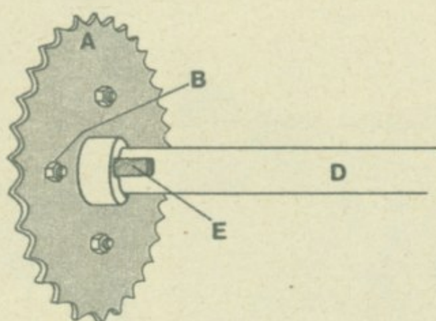
ЛАНЧАНИК (гледан из задњег десног угла): а) ланчаник, б) шраф, с) осигурач осовине, д) погонска осовина.
