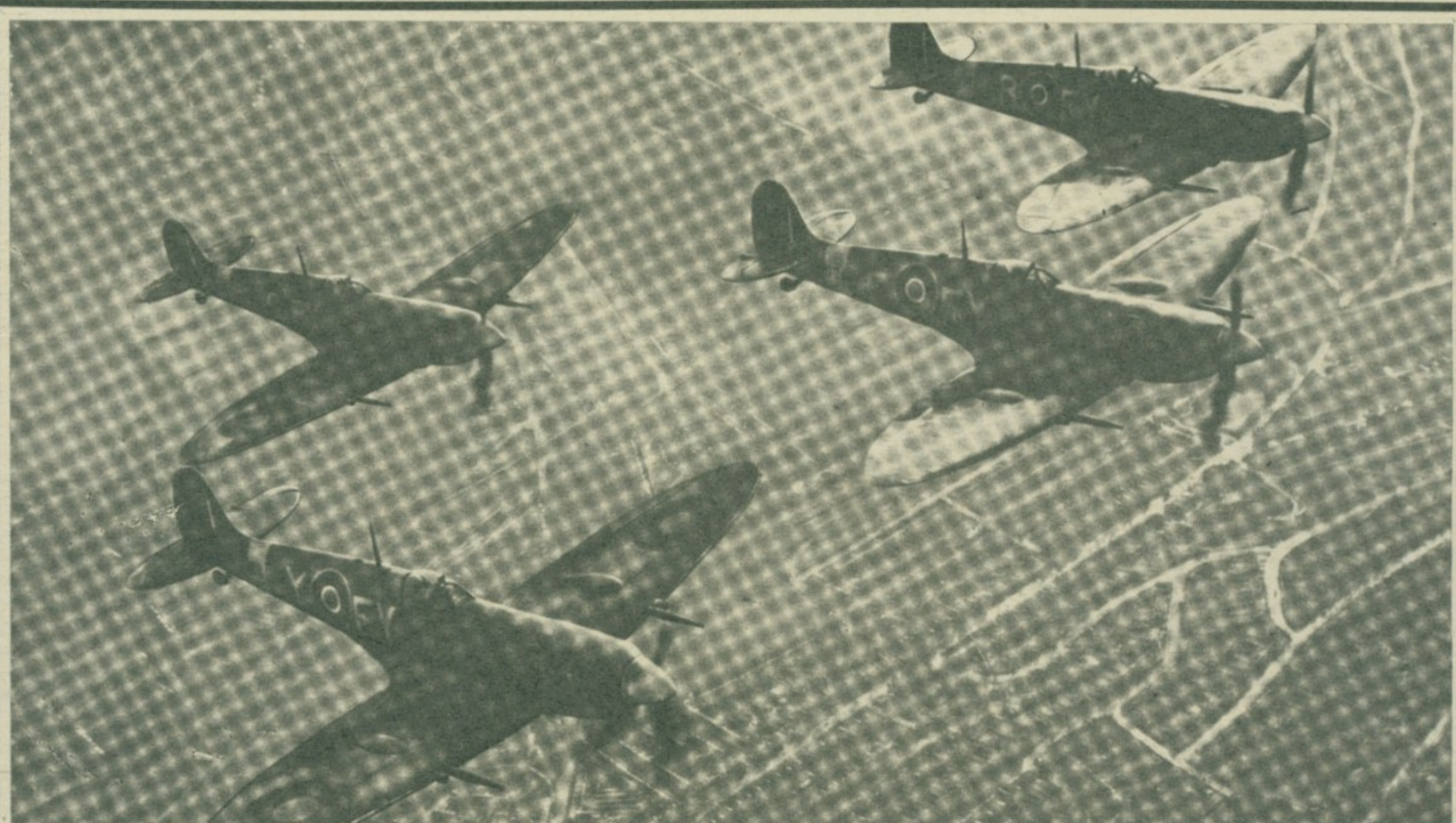
СПИТФАЈЕР: ловац једносед, металне конструкције, једнокрилац. Мотор ролс-ројс мерлин од 1.175 КС за прву верзију. Касније мотор грифон од 2.000 КС чија је брзина 724 км/час. Распон крила 12 м, дужина 9,80 м, тежина празног апарата 2.500 кг, оптерећеног 3.100 кг. Доплет 1.800 км. Осам митраљеза калибра 7,9 мм.
