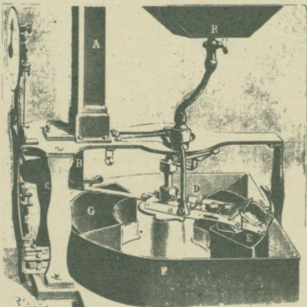
УНУТРАШЊИ МЕХАНИЗАМ ФЕРЕРОВОГ АПАРАТА
