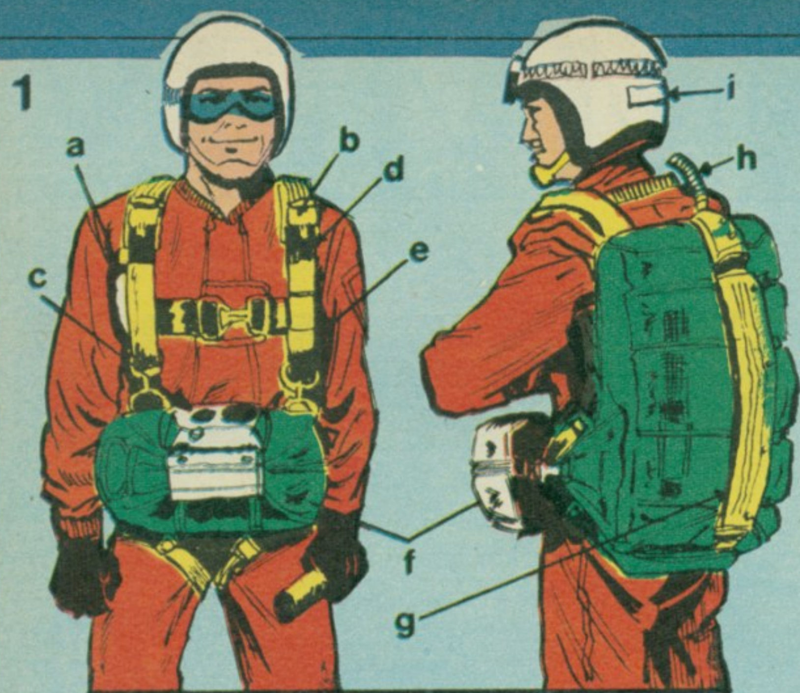
ОПРЕМА ПАДОБРАНЦА — а) ручица за активирање падо- брана; б) уређај за одбацавање куполе са конопцима; в) што- перица; д) систем веза; е) висиномер; ф) резервни падобран; г) поклопац за затварање ранца падобрана; х) гипко црево за сајлу која отвара падобран; и) кацига.
