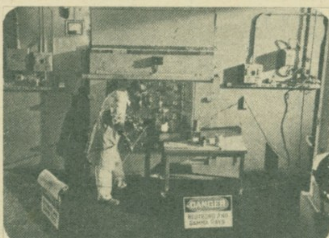
ЈЕДАН ГРАМ РАДИЈУМА ЕМИТУЈЕ ЗА ЈЕДАН СЕКУНД 3,7 МИЛИЈАРДИ АЛФА-ЧЕСТИЦА!
