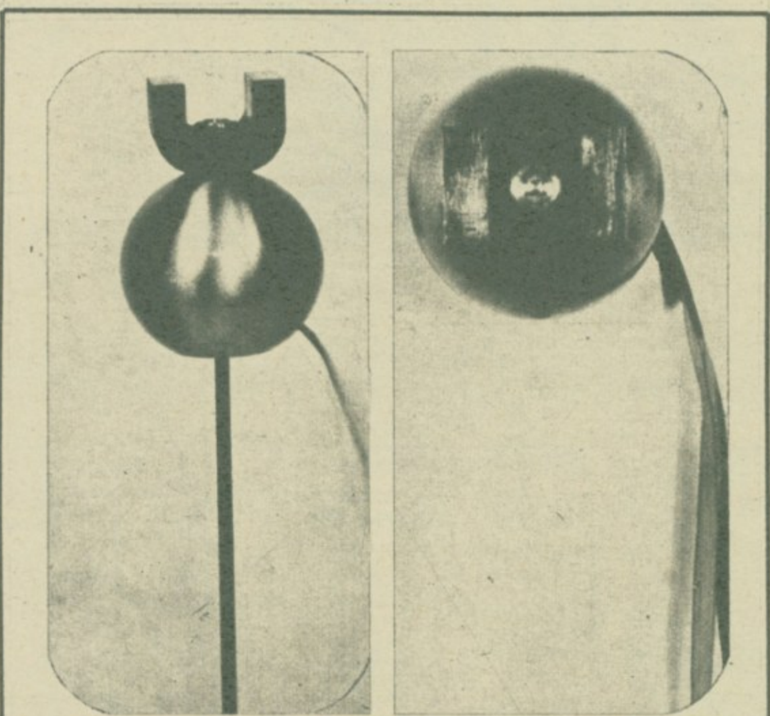
САВРЕМЕНА РЕКОНСТРУКЦИЈА ПРАСТАРОГ КОМПАСА: МЕТАЛНИ СТОЈЕР, ШУПЉА КУГЛА И ПОТКОВИЦА КОЈУ МАГНЕТИШЕ КОМАД ПРИРОДНОГ МАГНЕТА. НА СЛИЦИ ДЕСНО ЈАСНО СЕ ВИДИ КОМАД КАМЕНА КОЈИ МАГНЕТИШЕ ПОТКОВИЦУ
