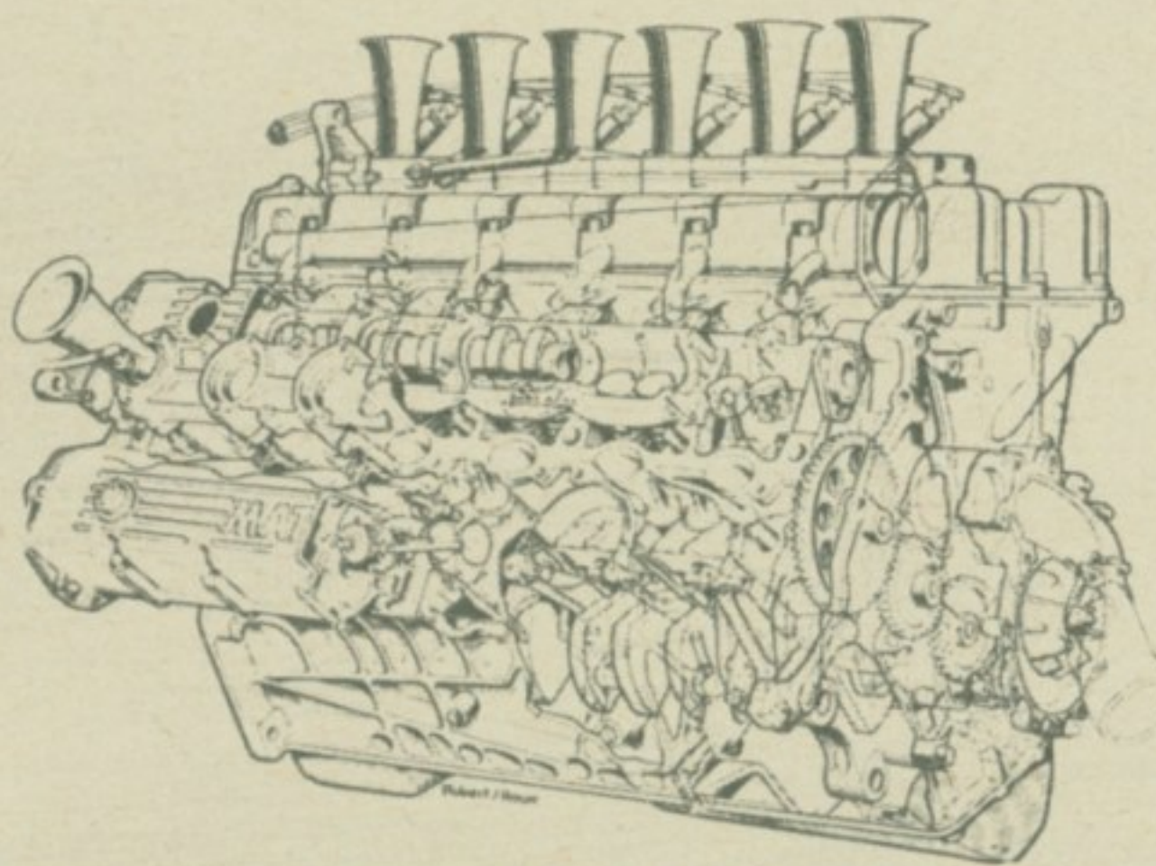
Овако изгледа мотор „матре“. На сваком, од укупно 12 цилиндара, налазе се по 4 вентила.
