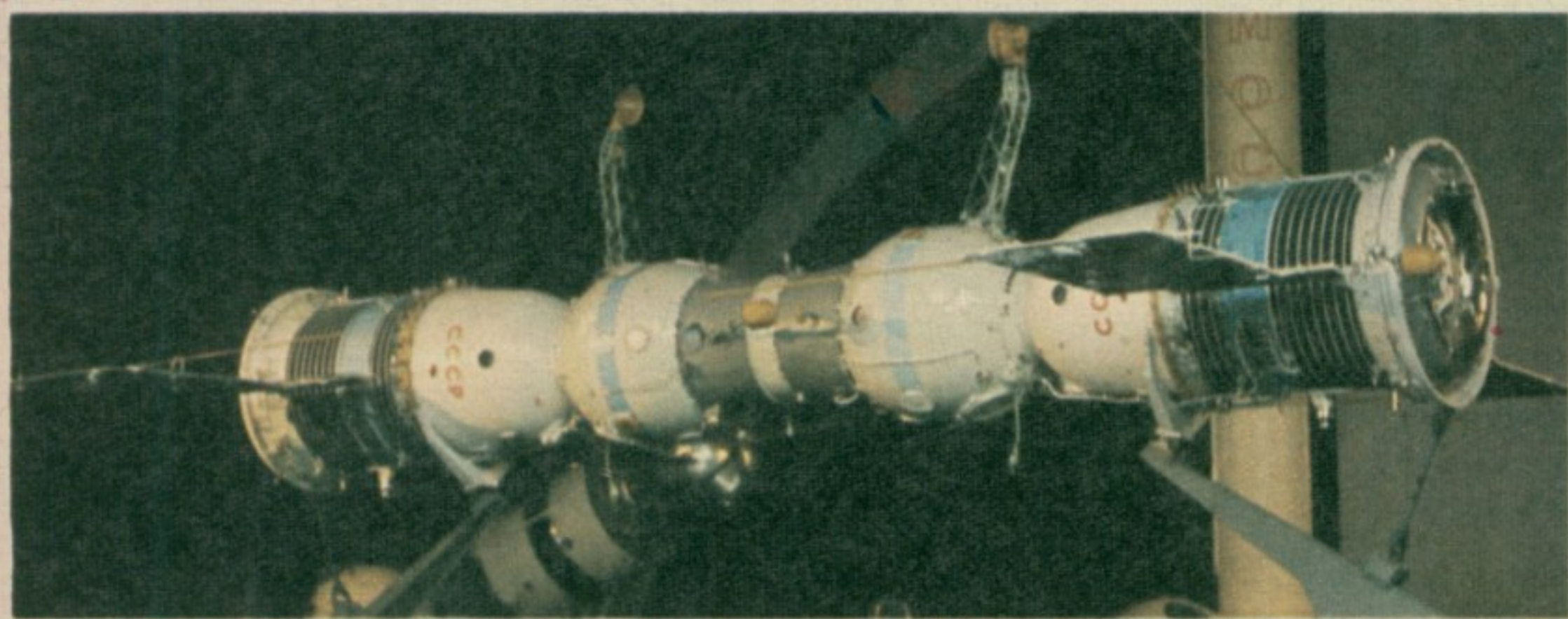
Прва експериментална орбитална станица СОЈУЗ настала је спајањем два брода СОЈУЗ 4 и СОЈУЗ 5 у васиони.
