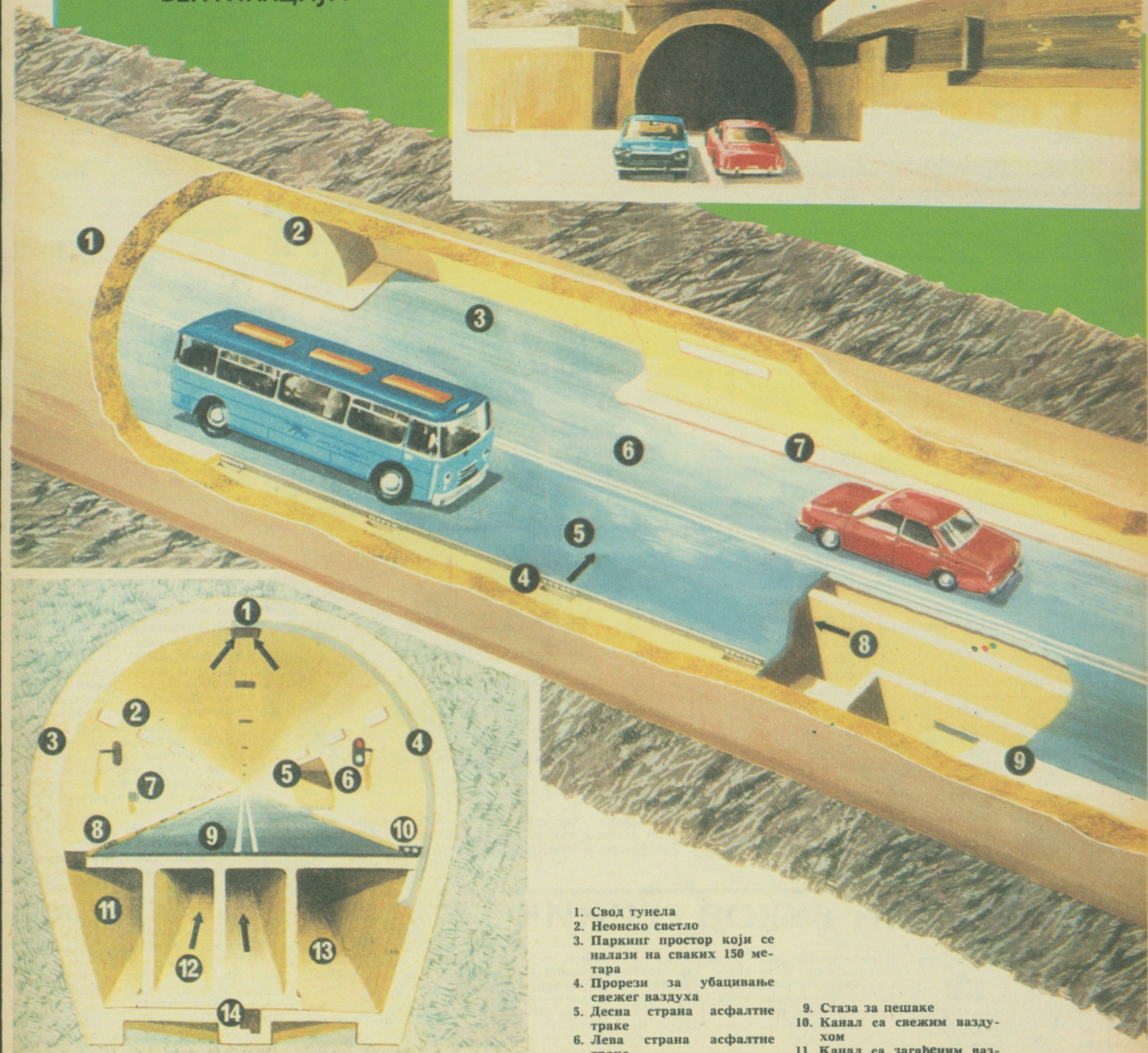
ПОПРЕЧАН ПРЕСЕК КРОЗ ТУНЕЛ
