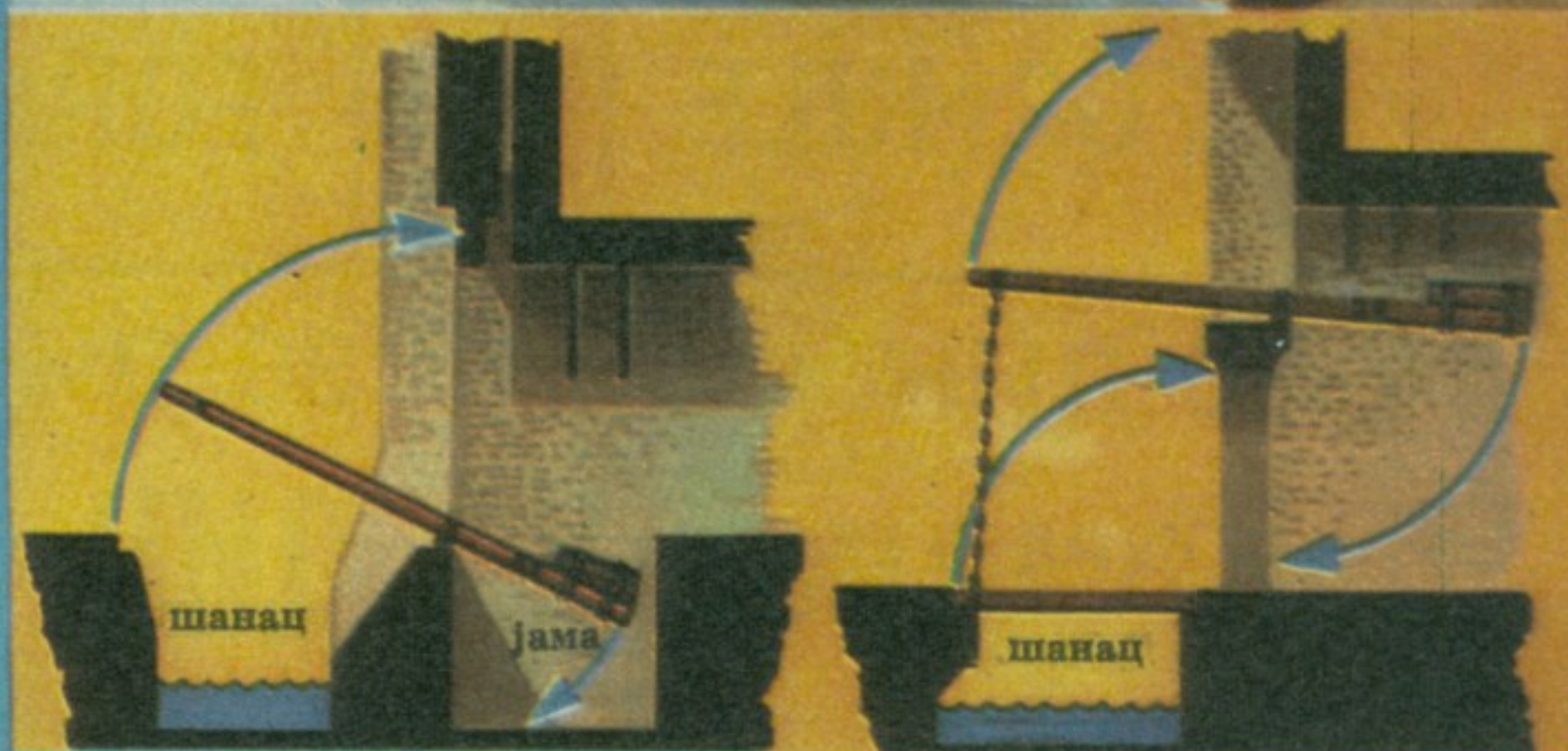
Два начина за подизање покретног моста: (А) За један крај моста причвршћен је терет који га вуче надоле, у посебну јаму (В) Подизање моста врши се уз помоћ греде која се налази изнад њега. Мост и греда повезани су ланцем.
