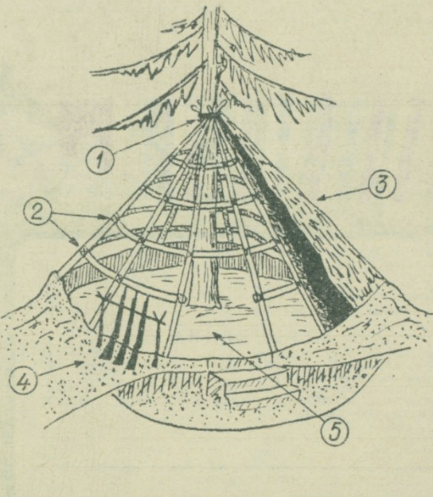
Округла колиба од грања везана за стабло: 1. Жица или конопца 2. Поплет 3. Грање наслањено наоцреп 4. Место за смештај хране, наоружања, опреме 5. Лежајеви подигнути слојем ситног грања (оно 30 см) прено којих се постављају папир и шаторска крила.
