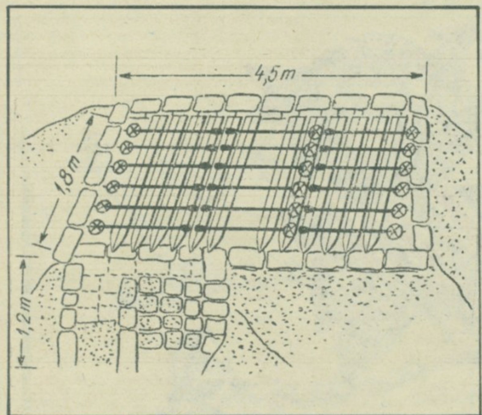
Начин израде снежне кућице
