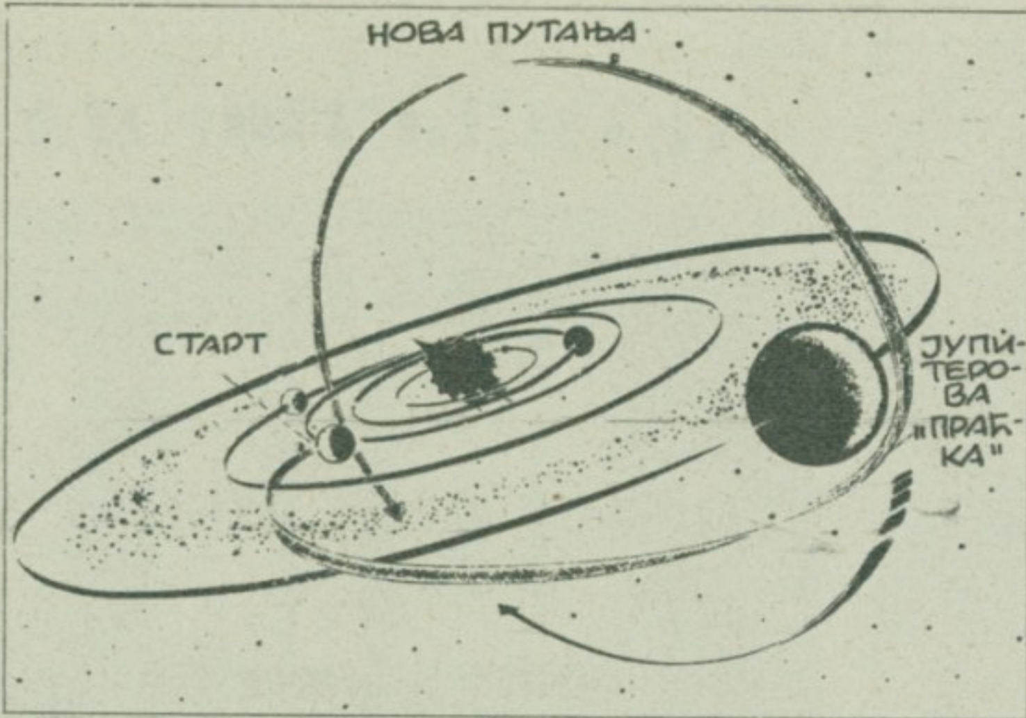
ЈУПИТЕРОВА ГРАВИТАЦИОНА СИЛА ОДБАЦУЈЕ ОБЕ СУНЧЕВЕ СОНДЕ И УПУЂУЈЕ ИХ НОВОМ ПУТАЊЕМ КА СУНЦУ.
