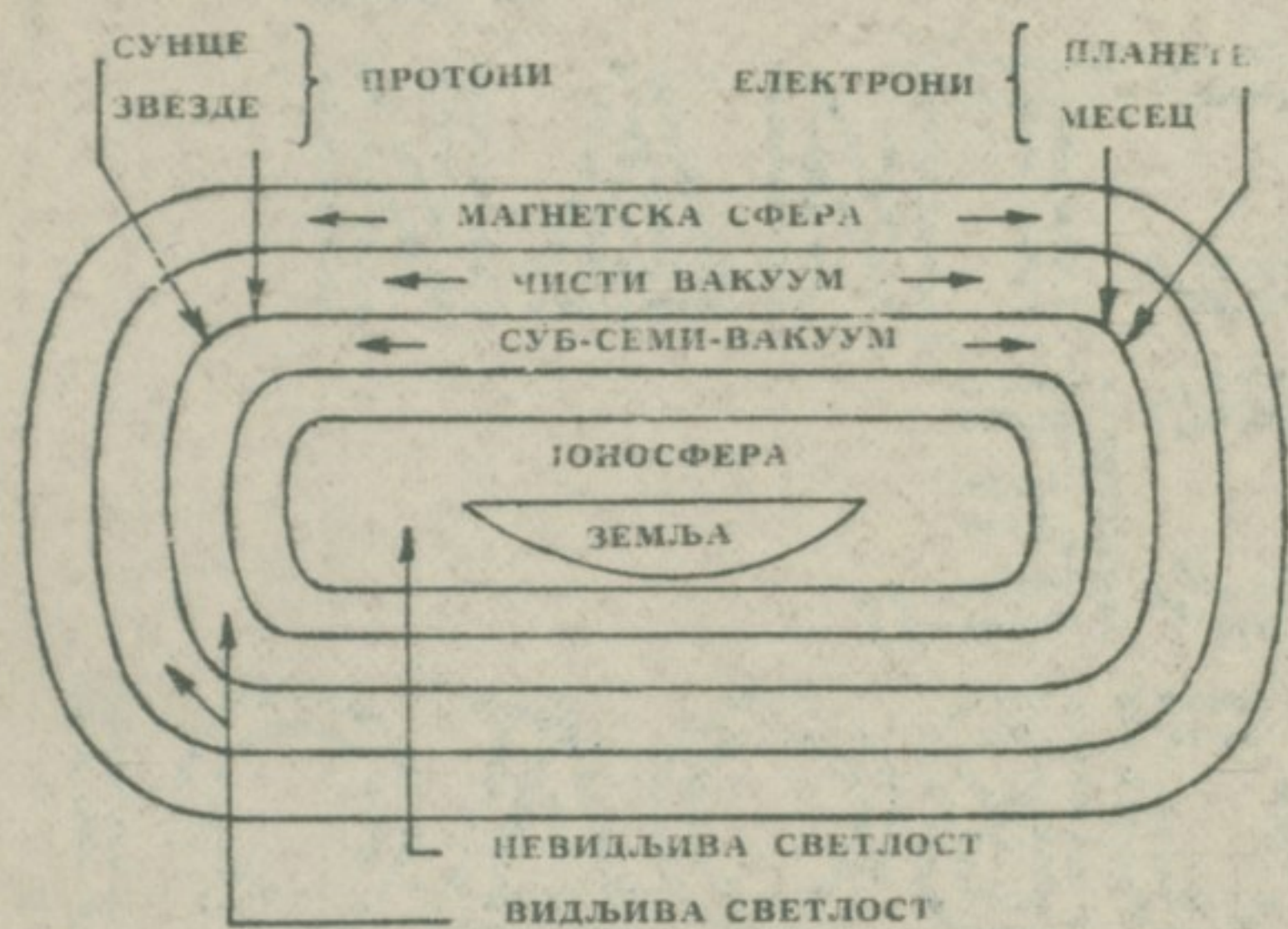
Шема свемира господина Бредберија
