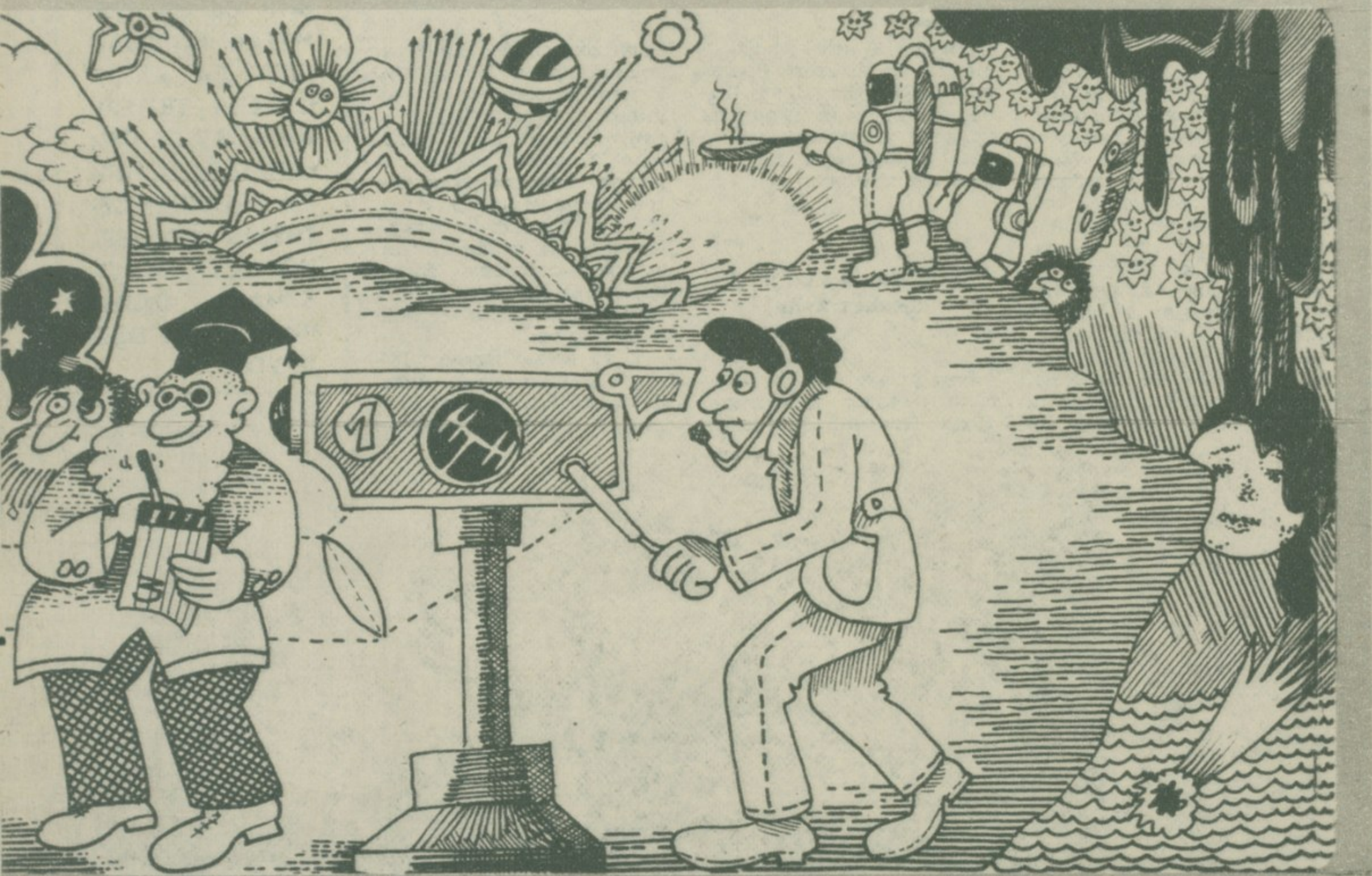
Шема свемира господина Бредберија
