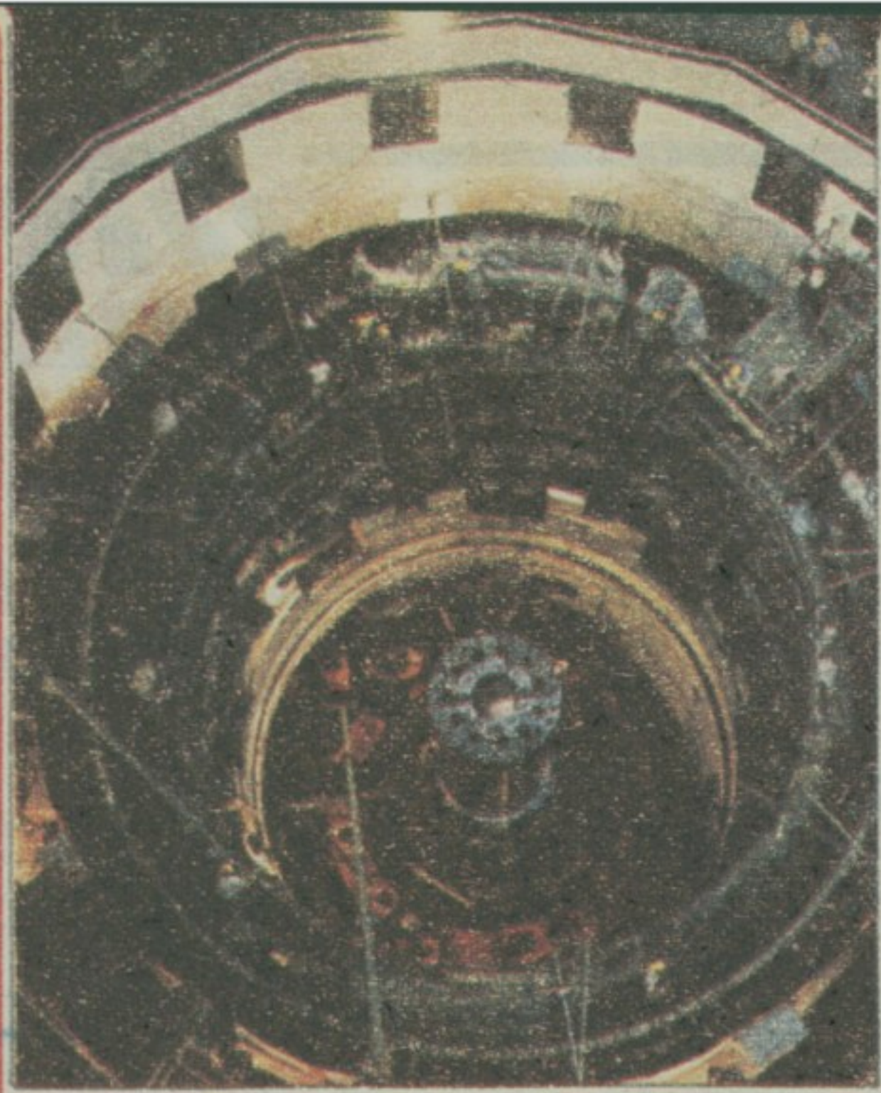
Огромни генератори пречника 20 метара
