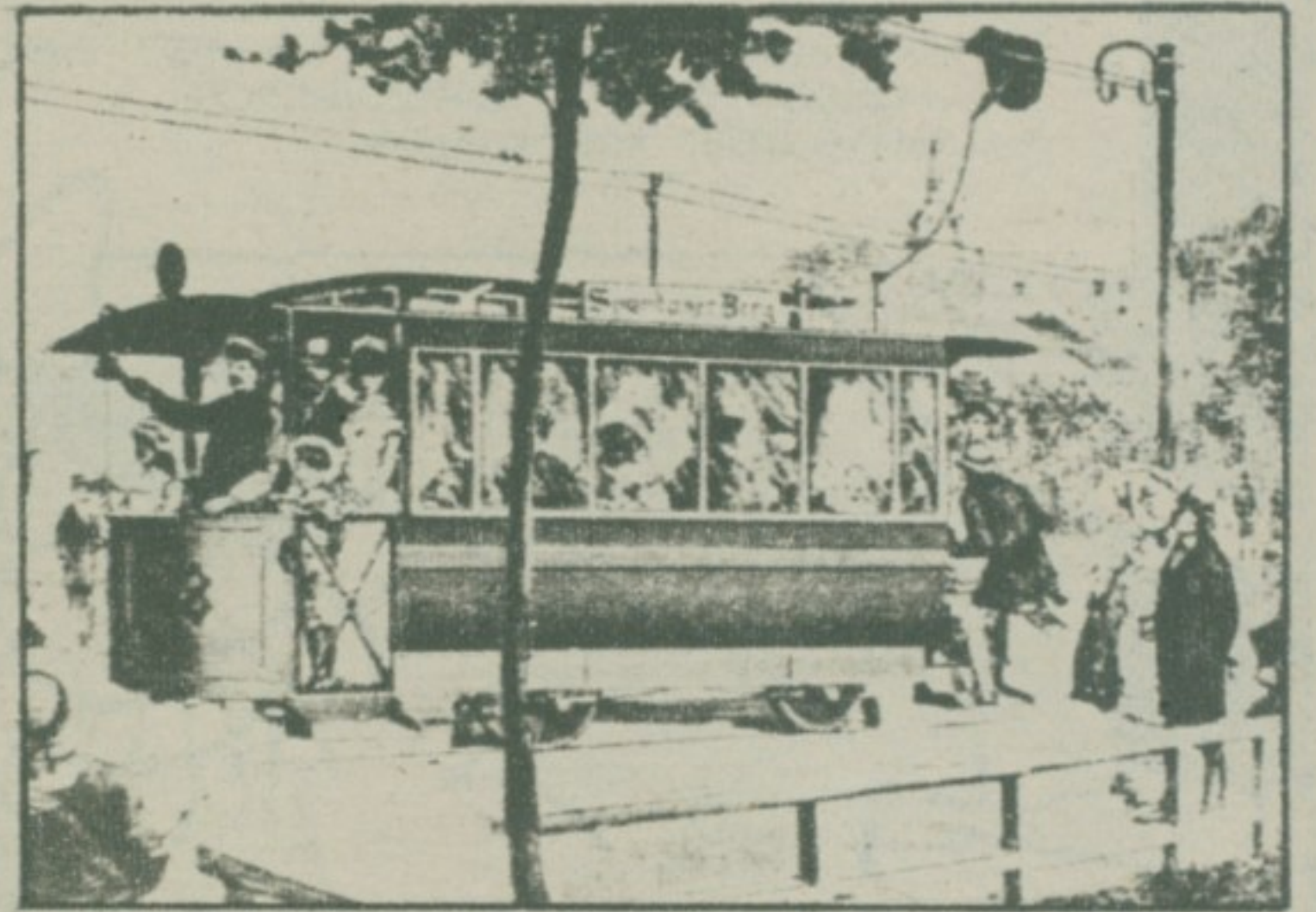
Први електрични трамвај на свету, дело браће Сименс, прошао је улицама Берлина 1882. године.
