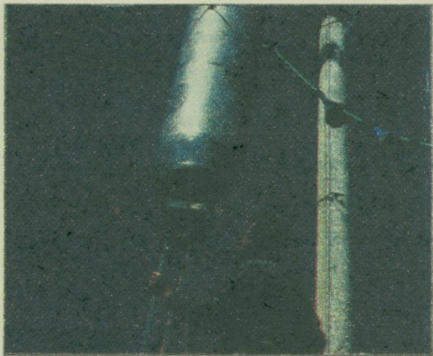
Алуминијумски цилиндар дуг десетак метара повезан је за торањ. То је „лажни авион“, у ствари стална жртва вештачке муње на којој се испитују последице овако снажног струјног и топлотног удара.
