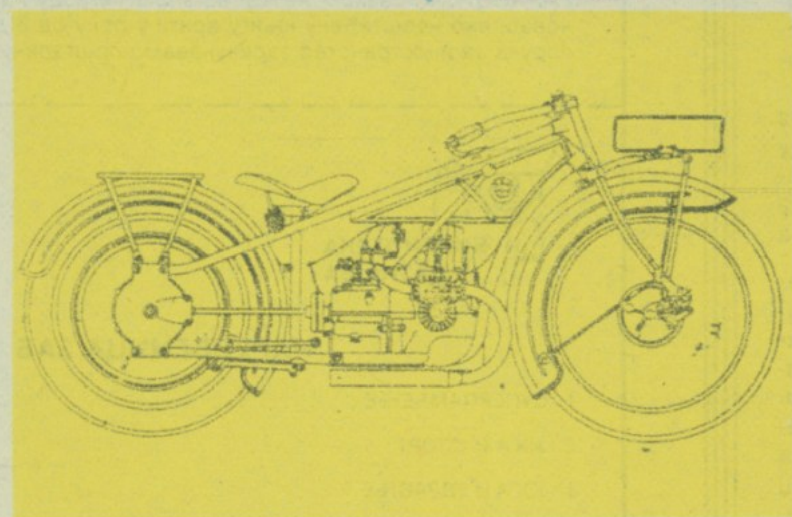
Технички цртеж првог BMW мотоцикла. Двоточкаш је носио ознаку R32 и дело је Макса Фрица. Цртеж се као светиња чува у дирекцији.
