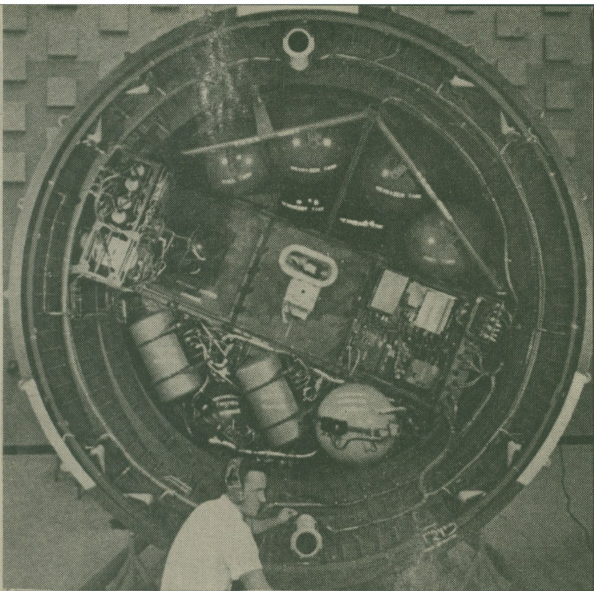
Део инсталација капсуле Џемини
