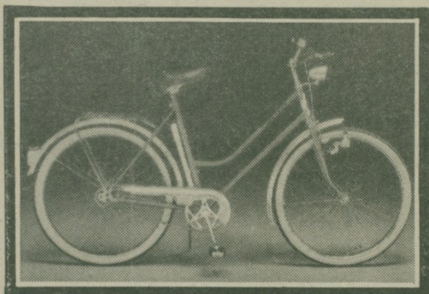
Бицикли женски „турист“, 28 цолова – 28 \times 1 \frac{1}{2} и 26 ц. – 26 \times 1 \frac{3}{8} . Рам је од шавних цеви, гуме жичане, глава са кочницом система „торпедо“. Цена 6 471.–, рата 1 078,50 дин.
