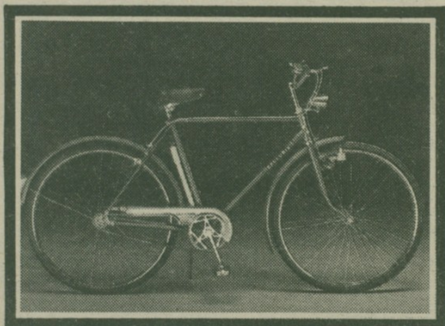
Бицикл мушки „турист“, 28 цолова – 28 \times 1 \frac{1}{2} и 26 ц. – 26 \times 1 \frac{3}{8} . Рам је од шавних цеви, гуме жичане, глава са кочницом система „торпедо“. Цена 6 471.–, рата 1 078,50 дин.
