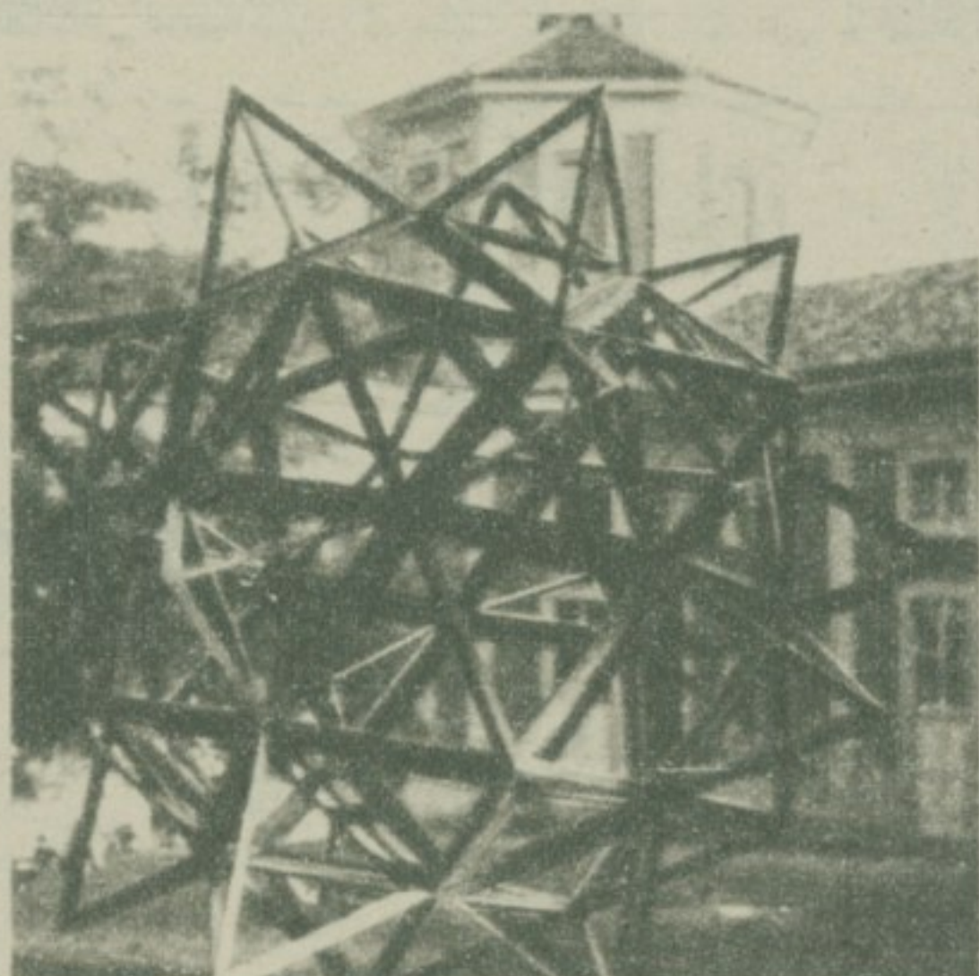
Леонардов полиедар. Кад је замољен да га нацрта, Да Винчи, кажу, није имао појма о геометрији.
