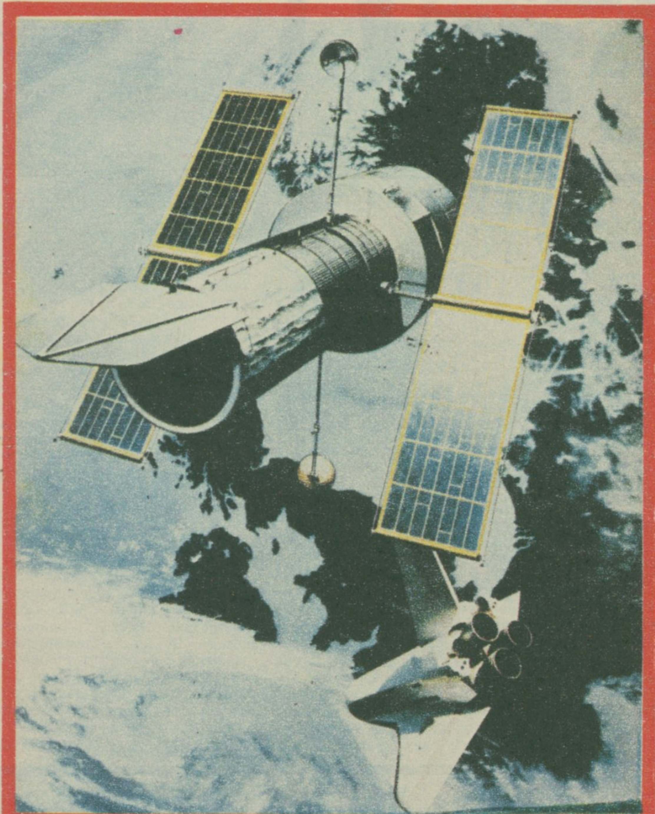
Свемирски телескоп британске фирме „Бритиш Аероспејс“, који ускоро треба да буде избачен у орбиту, можда ће открити планете изван Сунчевог система.
