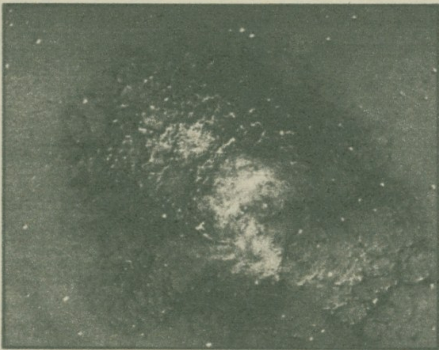
Експлодирало сунце (супернова у сазвезђу Бик) снимљено два пута у размаку од 14 година: фотографије експлозивних облака су унопиране једна преко друге, чиме је добијен пластичан утисак покрета комадића облака. Људи су овај догађај посматрали 1054. године – а облаци се још увек разилазе брзином од 1.100 километара у секунди.
