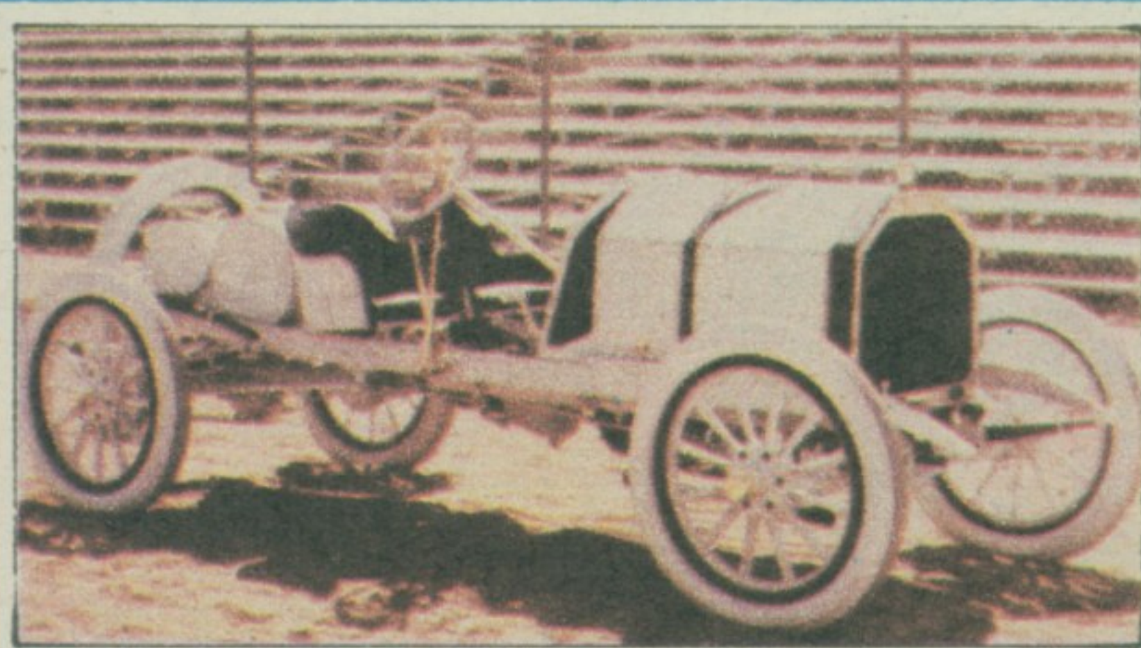
1910. Буик Рејсер. Дејвид Буик је хтео да тржишту понуди спортске аутомобиле. С овим четворцилиндрашем од 70 коњских снага Боб Барман је победио на првом такмичењу у Индијанаполису.
