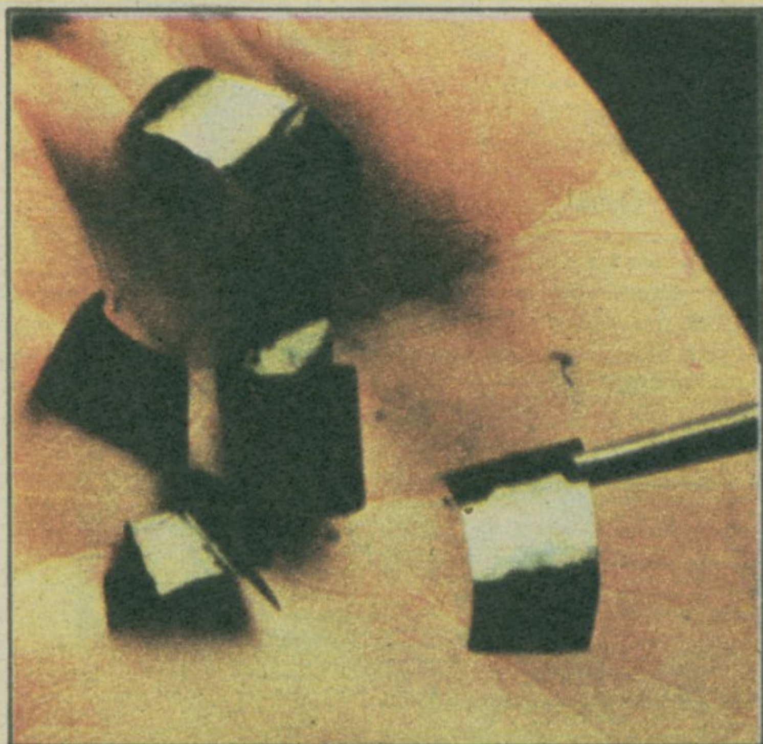
Листићи полиацетилена
