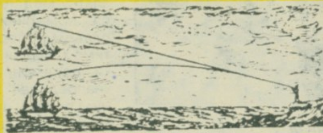
Две основне врсте опсена: „нижа опсена“ настаје у врућим пределима, када је доњи слој ваздуха топлији и ређи (горе) „Виша опсена“ јавља се у хладним подручјима, где доњи слој има нижу температуру и гушћи је (доле)
