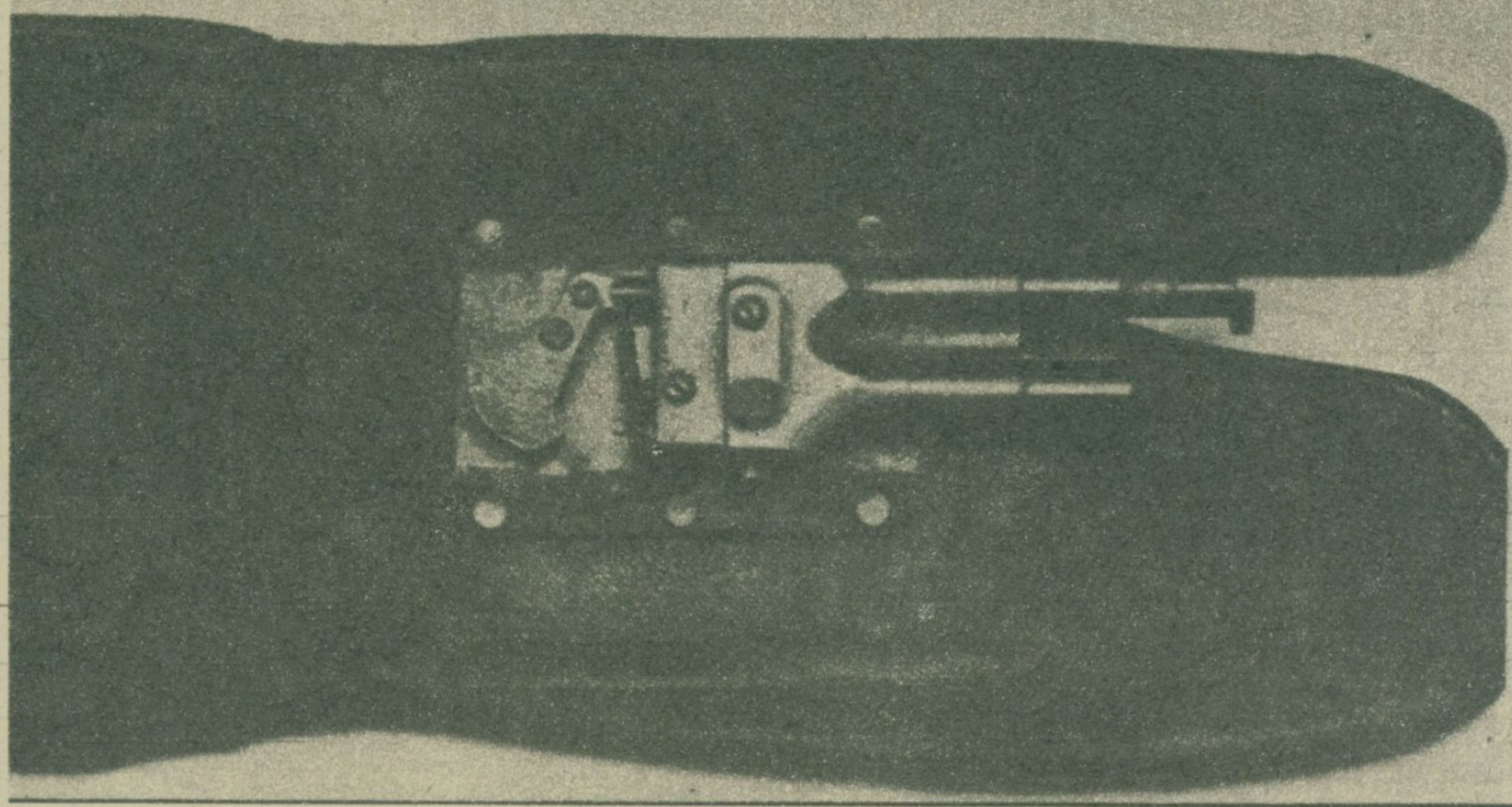
„Пиштољ-рукавица“ у серијској верзији: тип „МК-II“ са орозом
