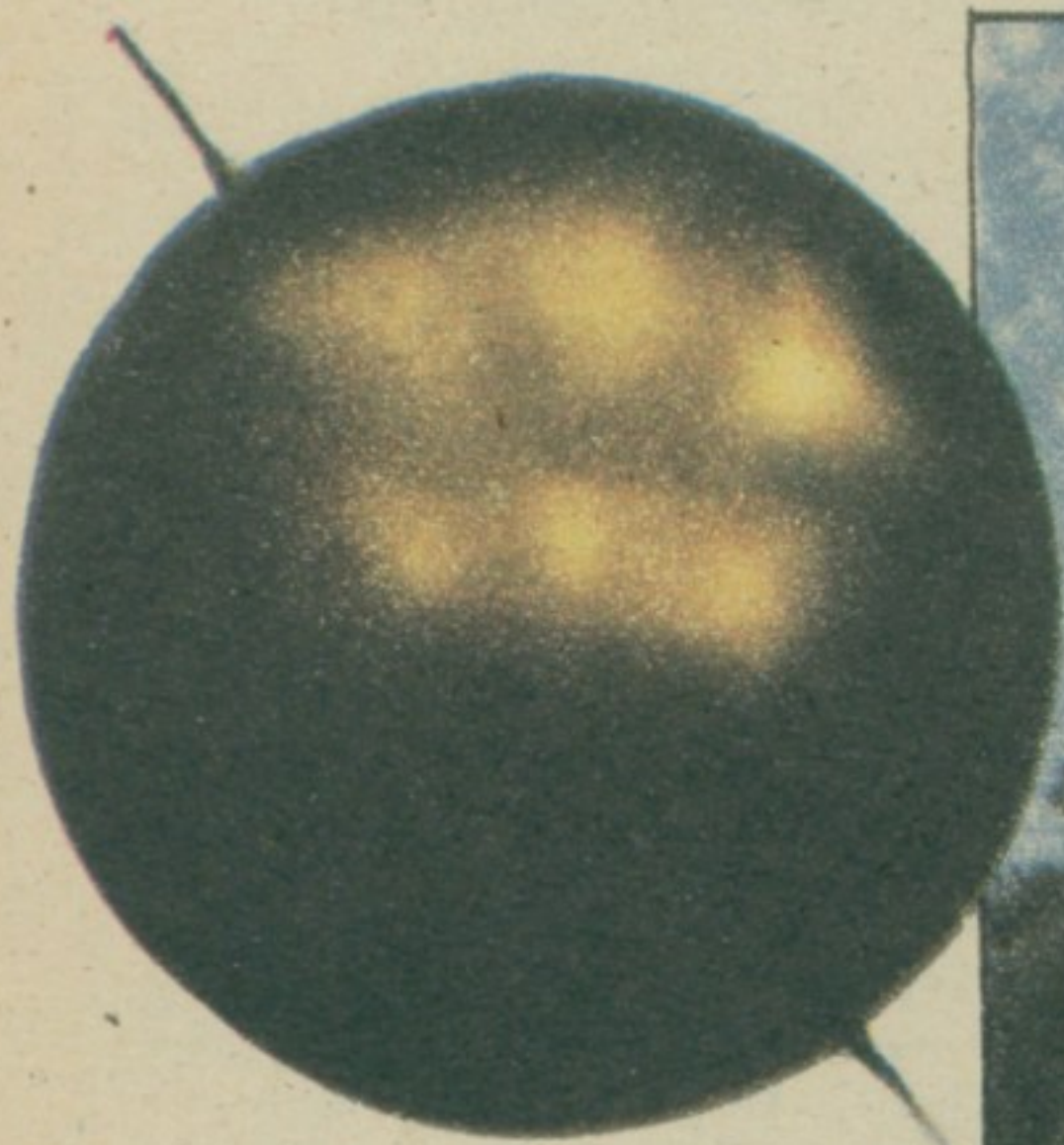
Тајанствена кугла: специјалиста за теоријску физику Питер Тајбергер камповао је на врху ове стене да би „осетио“ пету силу. Ова шупља бакарна лопта, пречника 20 центиметара, пливајући у води „помери“ се сама од себе неколико центиметара на сат
