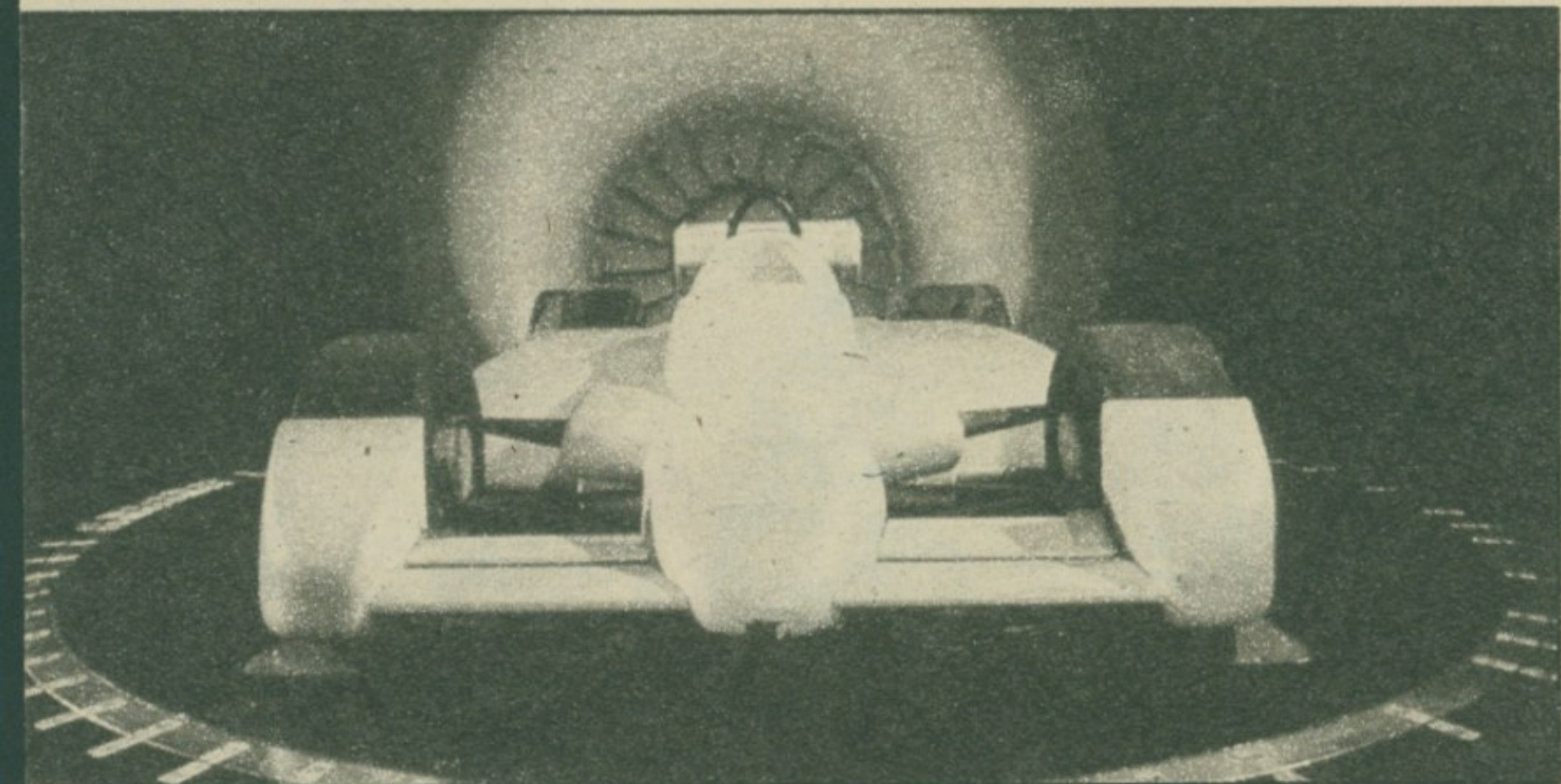
Модел једне од најновијих „формула 1“ спреман за оглед у Ајфеловој лабораторији.
