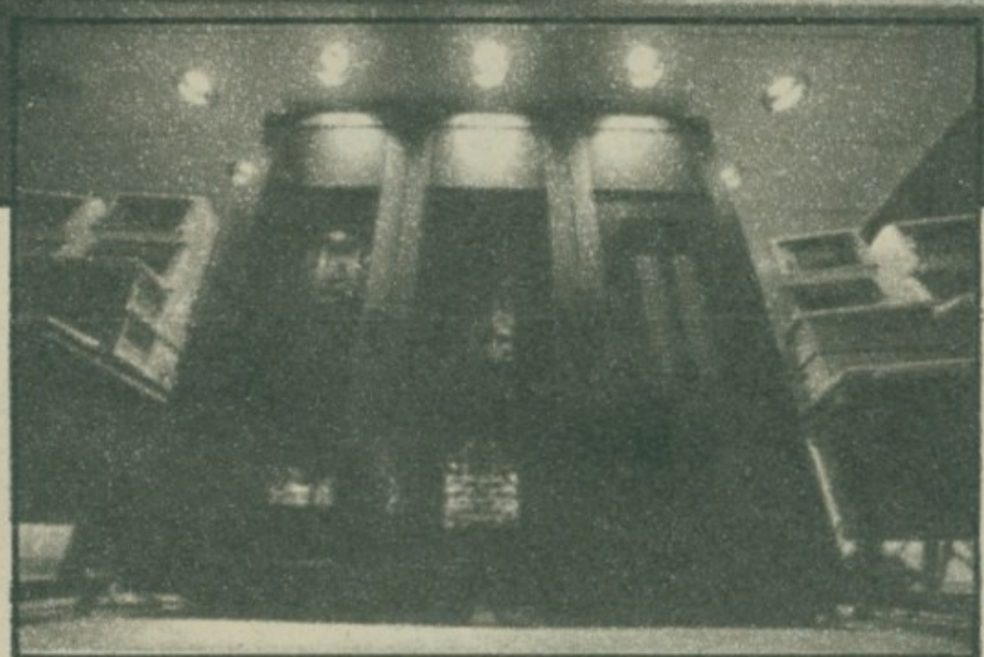
IBM је у Јорктауну направио нову генерацију ултра брзих чипова (горе) за паралелне компјутере као што је RP 3 (лево) са мрежом од 64 међусобно повезана микропроцесора. Следећа етапа: створити TF 1 који ће изводити 1500 милијарди операција у секунди.
