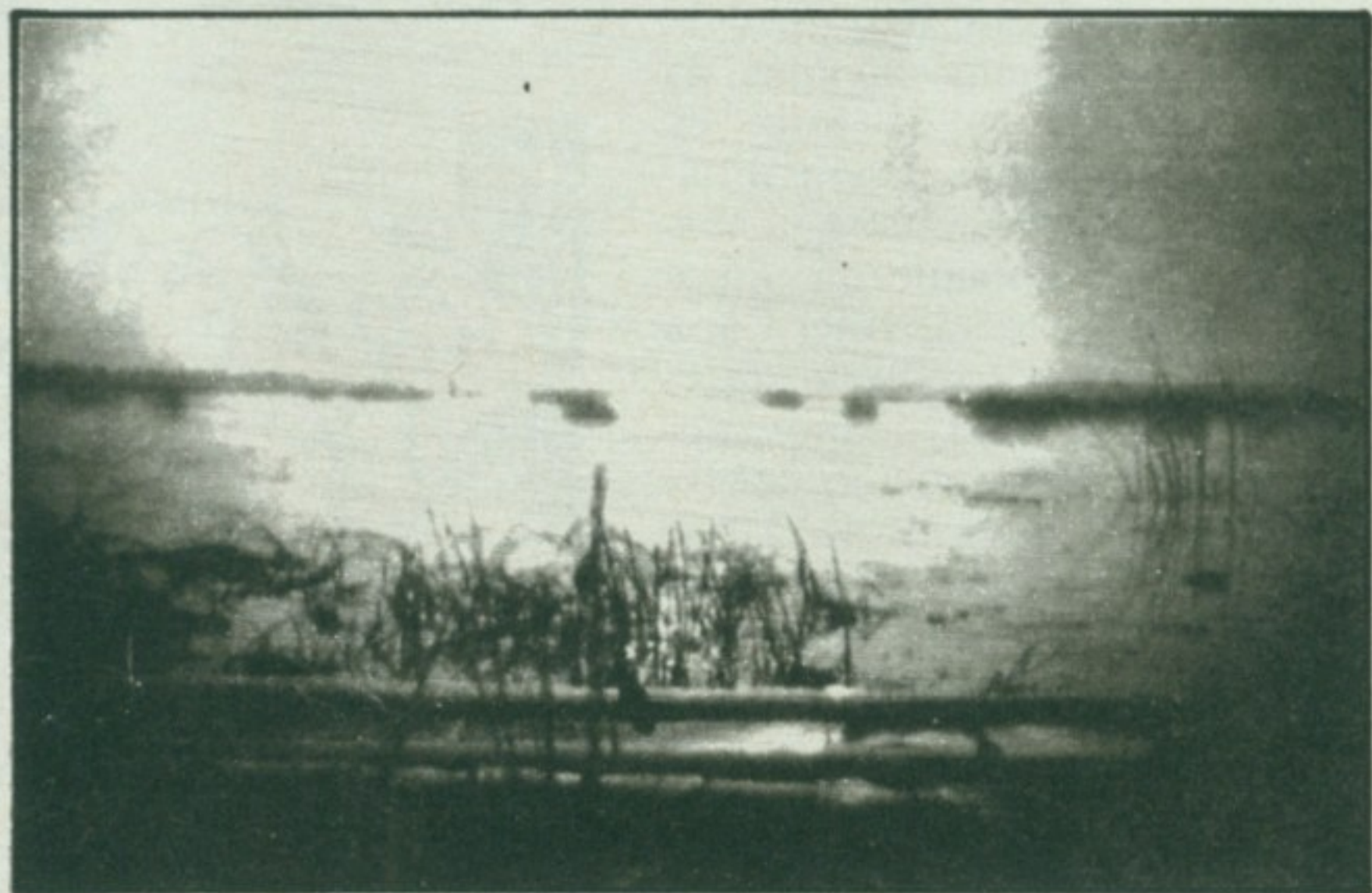
Трагови лоптасте муње која се појавила 22. августа 1986. на језеру Шид у Архангелској области
