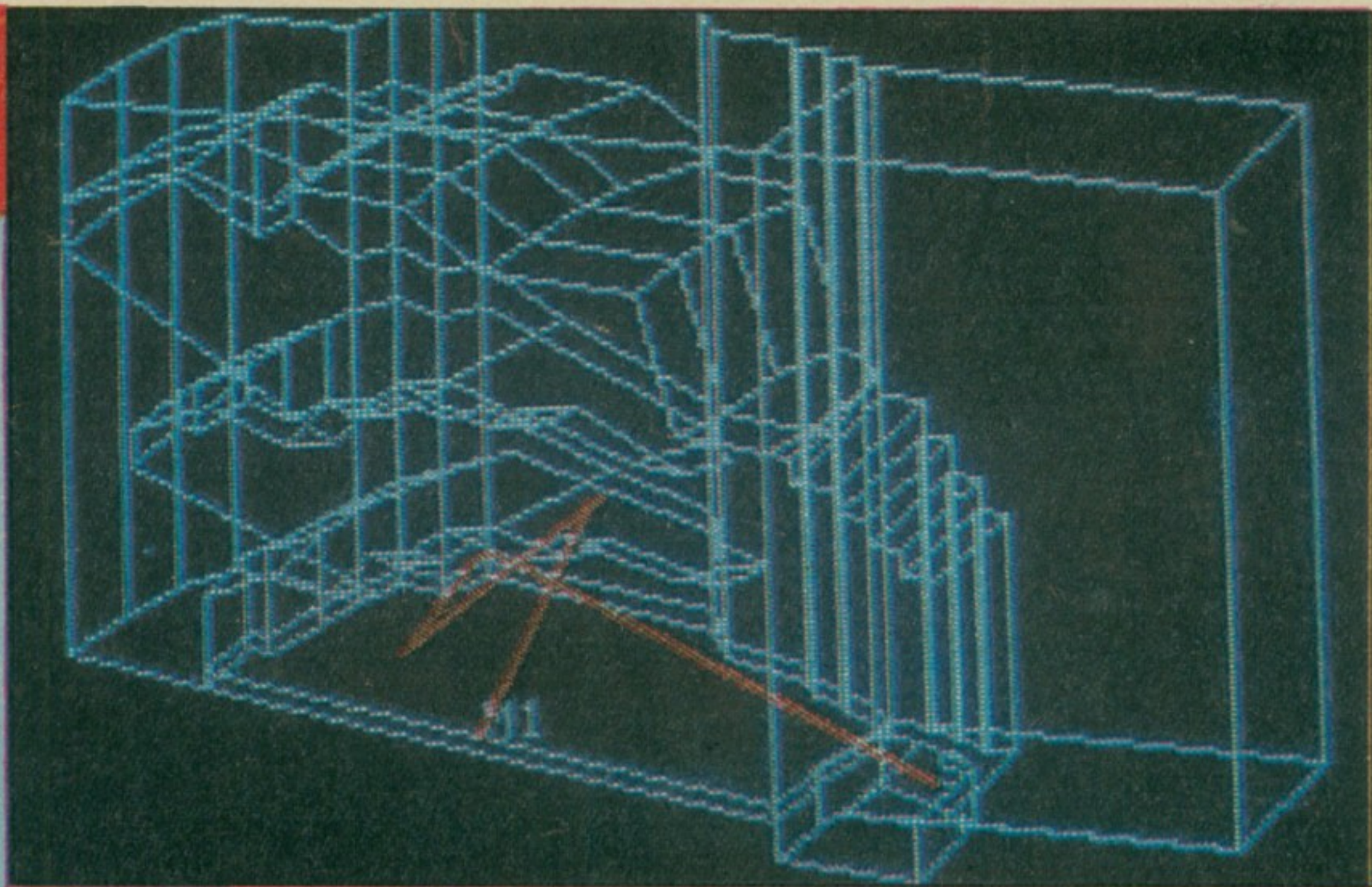
„НАЈДЕМОКРАТИЧНИЈИ“ ЗВУК. Звучне мапе направљене на симулатору показују путање звучних таласа (црвено) до сваког слушаоца у сали са 2700 места.
