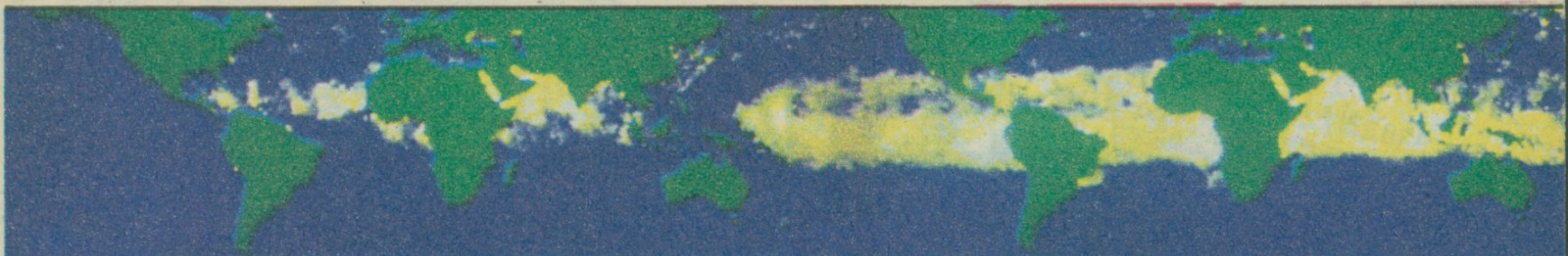
Сателитска слика ширења копрене вулканских честица после ерупције Пинатуба на Филипинима јуна 1991.
