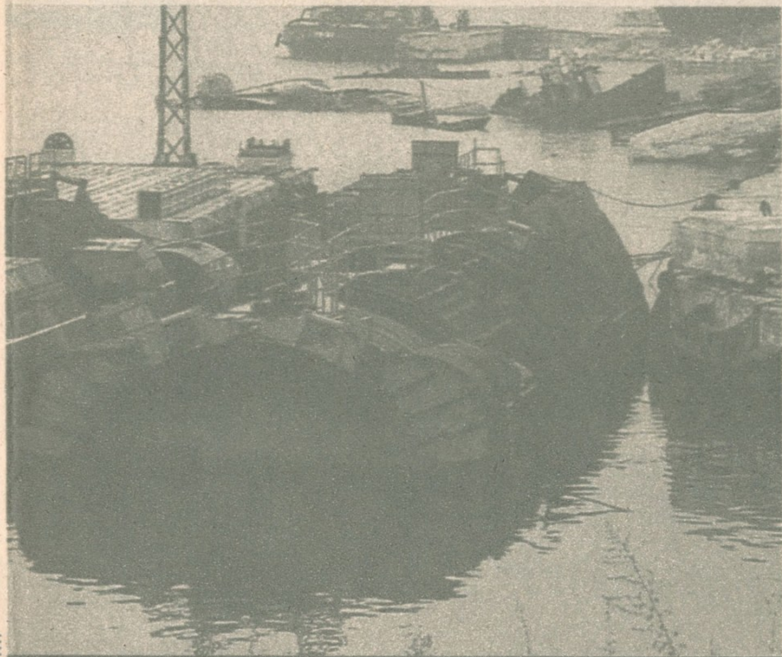
У заливу Чазма демантирају се руске „атомске“ подморнице које одлазе у старо гвожђе
