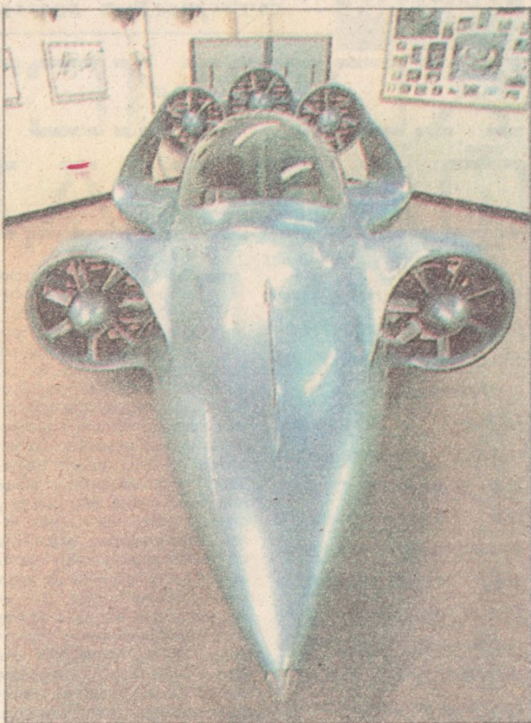
Прототип „М 400“: 1200 KS максимална брзина 650 km/h, а уз то још и лети.
