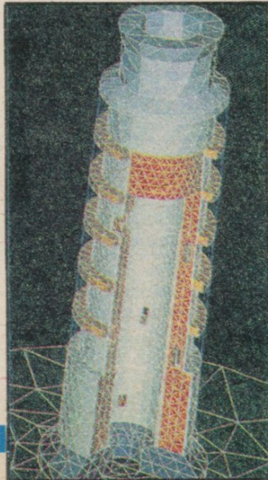
Компјутерска слика торња и модел једног од решења: стручњак је замислио да торањ притегне челичним сајлама!
