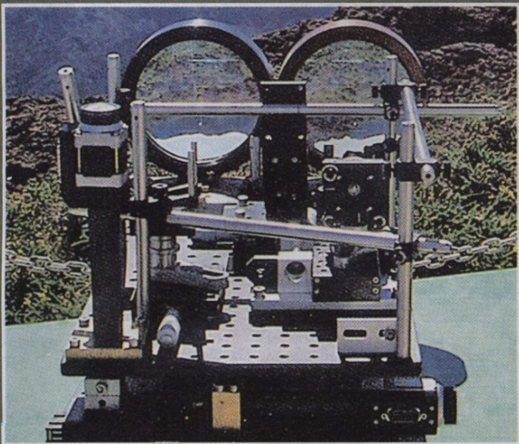
Телескопски предајник на Ла Палми уперен према пријемнику на острву Тенерифе. Једно од великих сочива преноси појединачне фотоне, док друго служи за одређивање тачног положаја, примајући ласерски зрак са другог острва.
